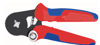
6060-030 Aderendhülsenzange - 0,08mm 2 bis 16mm 2 Aderendhülsen - Kraftverstärkung durch Kniehebel - Vierkantpressung für optimale Kontaktflächen in Klemmanschlüssen
